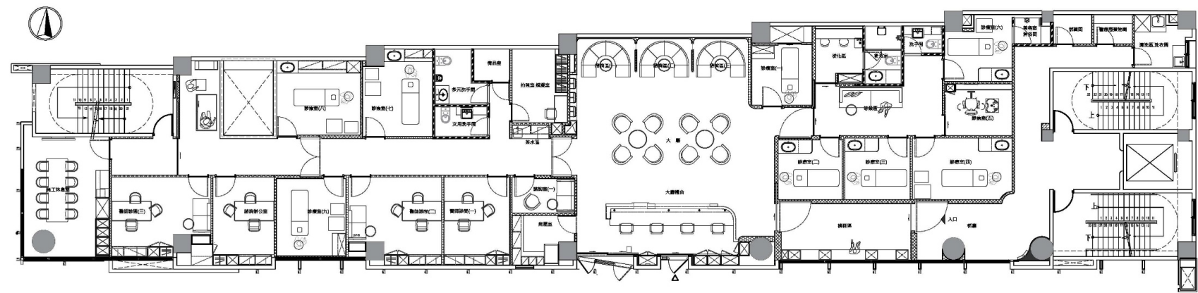
五樓 平面配置圖
