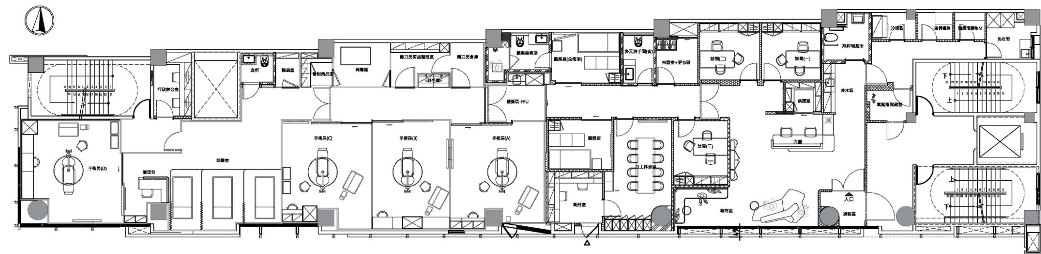
四樓 平面配置圖
