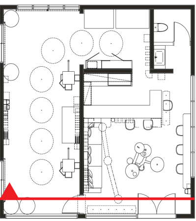
剖面A
