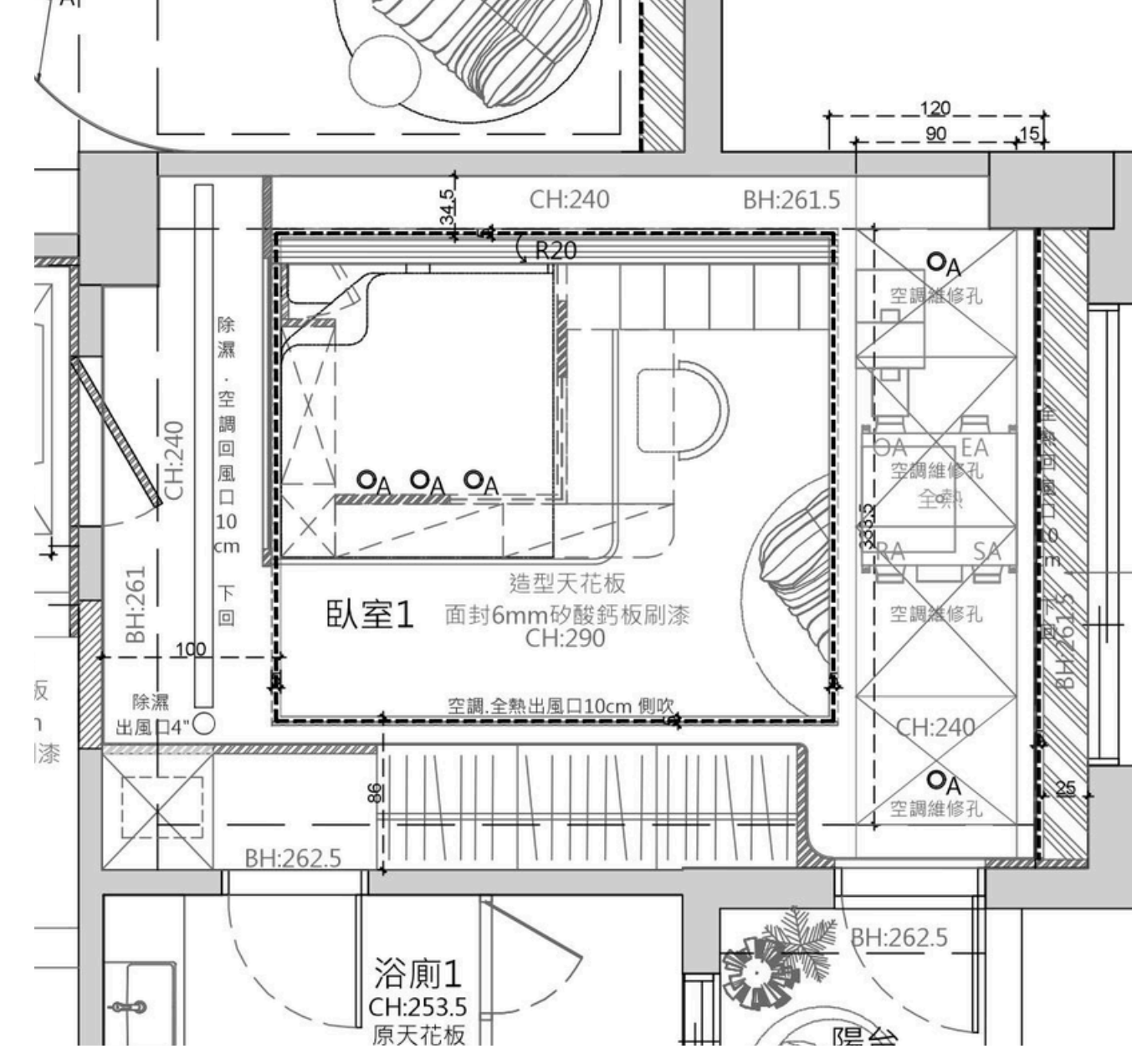
天花空調配置
