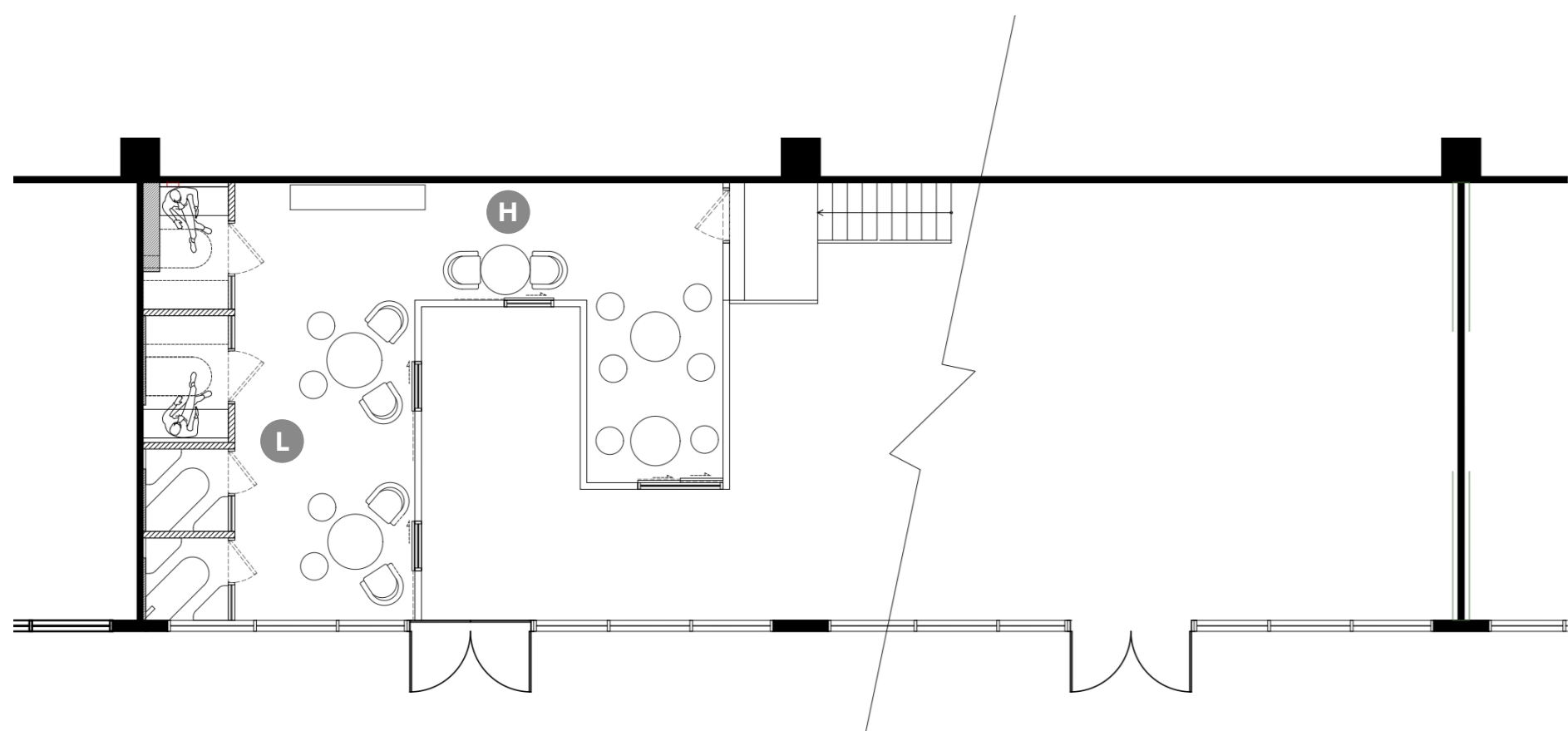
閣樓平面配置圖 MF Floor Plan.
