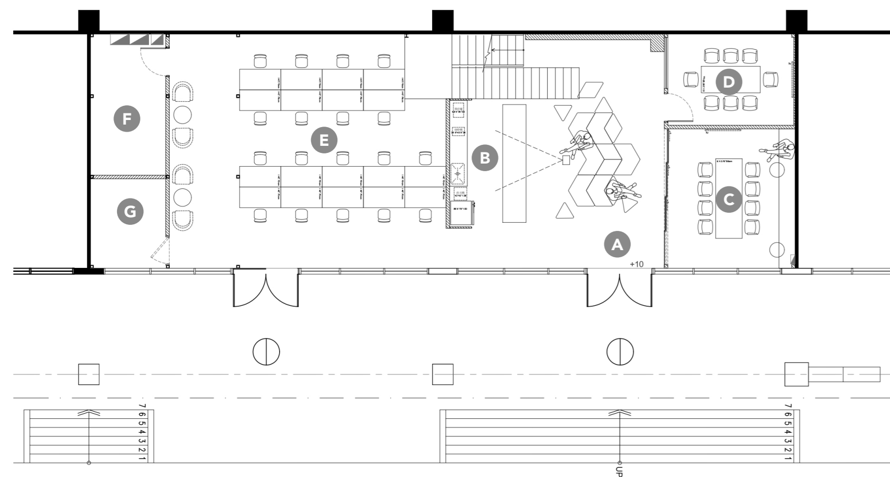
一樓平面配置圖 1F Floor Plan.
