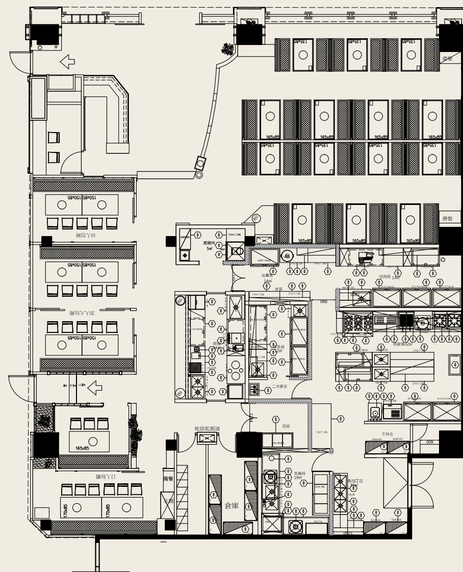
▲ 平面配置圖
