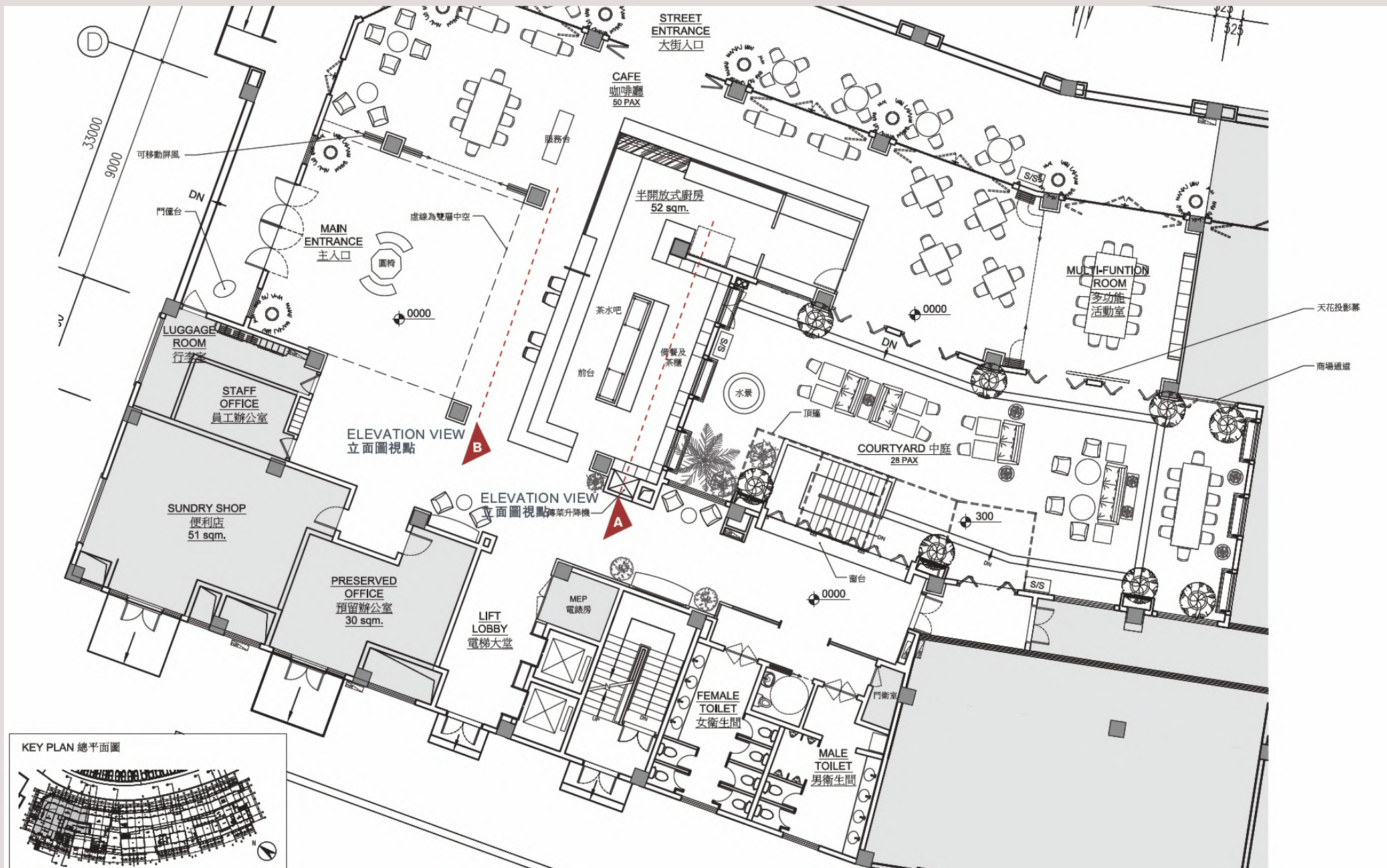
一層酒店大堂平面圖 HOTEL LOBBY FLOOR PLAN (LEVEL 1)
