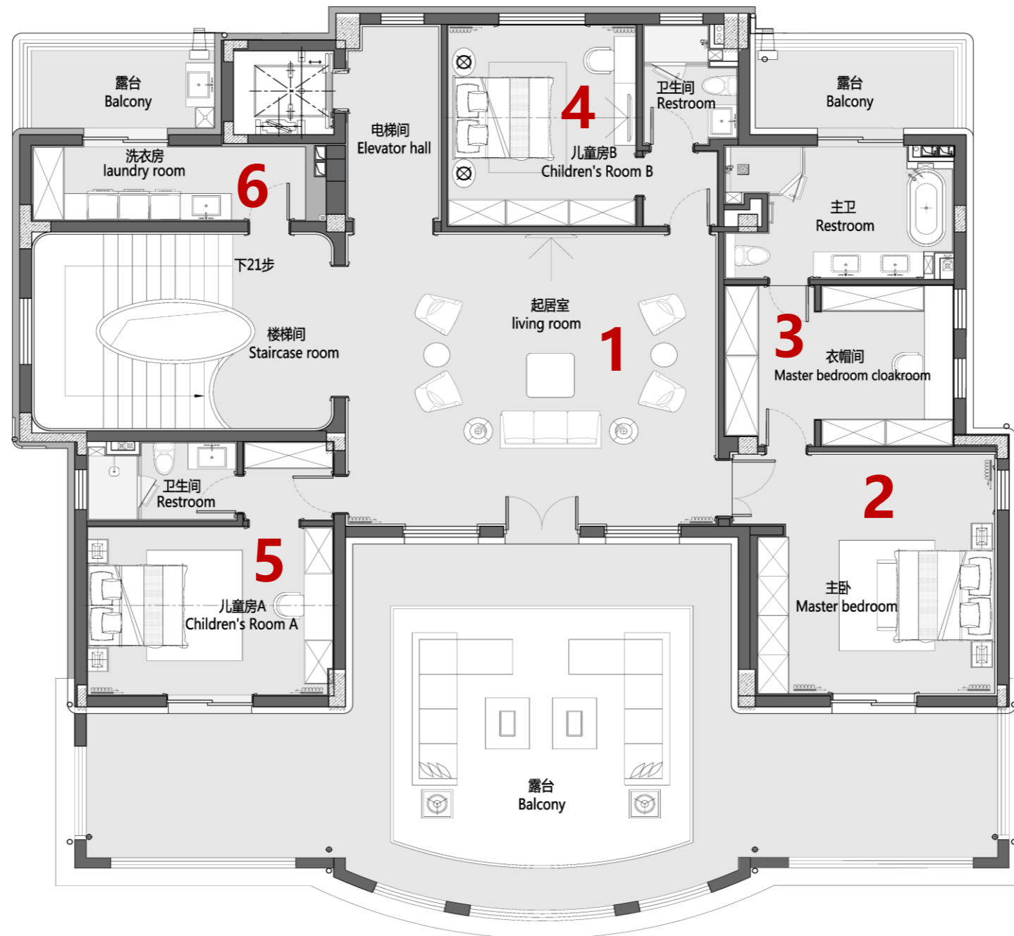
4F平面方案 4F floor plan
