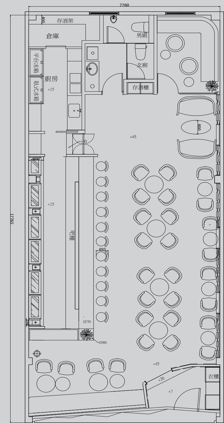
▲ 平面配置圖
